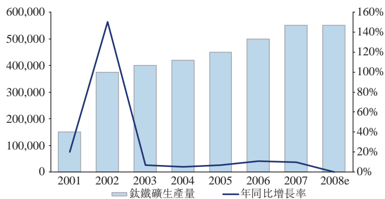
鈦鐵礦生產量(折算為二氧化鈦等價物，單位：噸)
